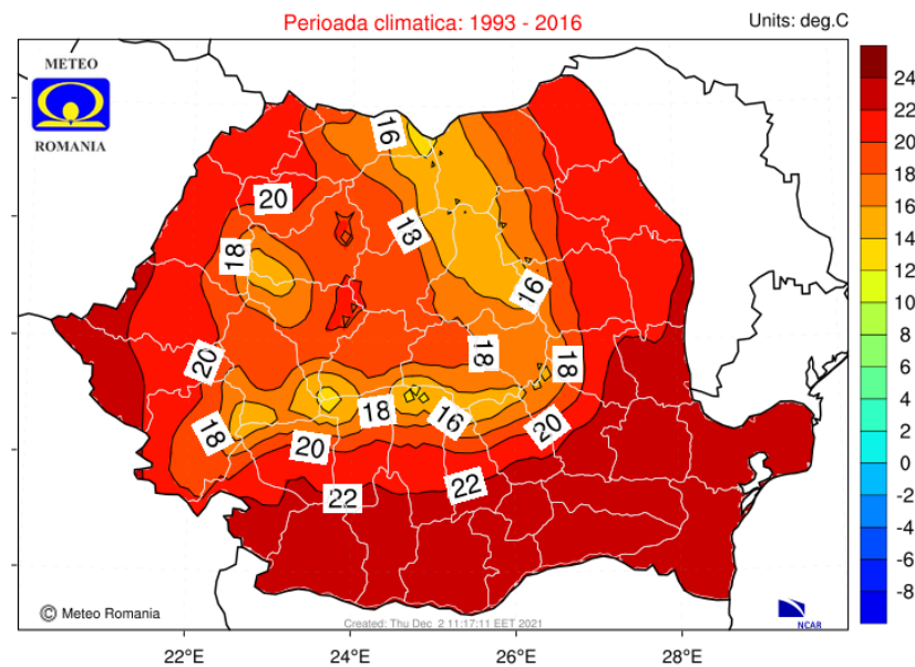
Temperatura aerului la 2m. Valori medii multianuale. Saptamana: 11/07 - 18/07
