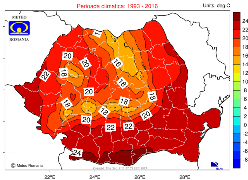
Temperatura aerului la 2m. Valori medii multianuale. Saptamana: 04/07 - 11/07
