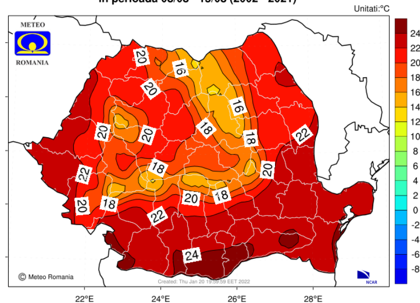
Media multianuala a temperaturii aerului la 2 m in perioada 08/08 - 15/08 (2002 - 2021)
