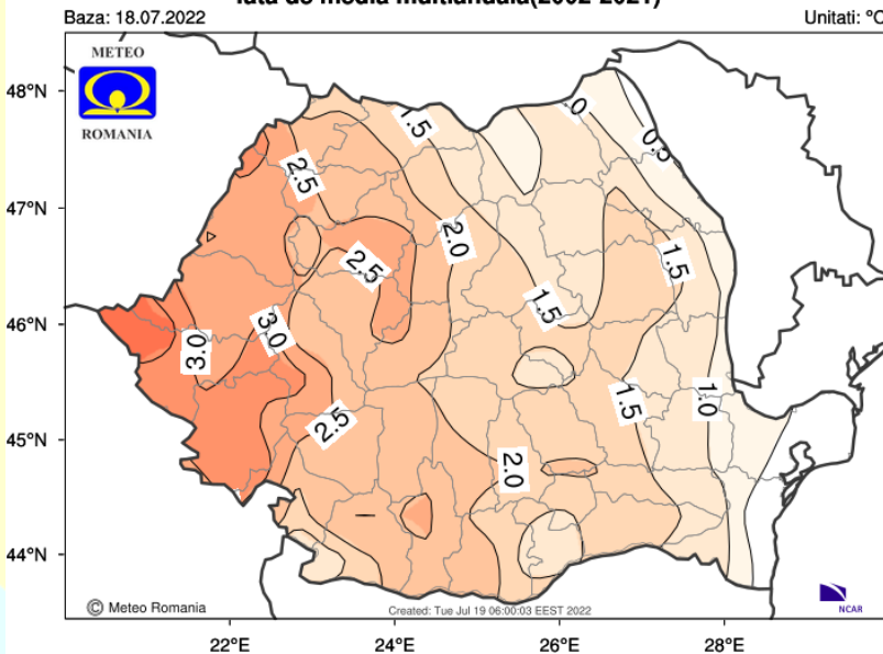
Abaterea temperaturii medii a aerului in perioada 18/07/2022 - 25/07/2022 fata de media multianuala(2002-2021)
