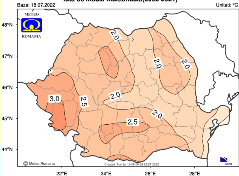
Abaterea temperaturii medii a aerului in perioada 08/08/2022 - 15/08/2022 fata de media multianuala(2002-2021)
