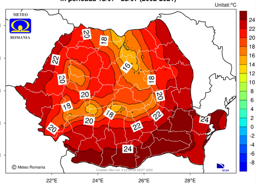
Media multianuala a temperaturii aerului la 2 m in perioada 18/07 - 25/07 (2002-2021)
