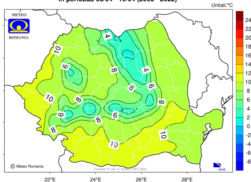
Media multianuala a temperaturii aerului la 2 m in perioada 03/04 - 10/04 (2003 - 2022)
