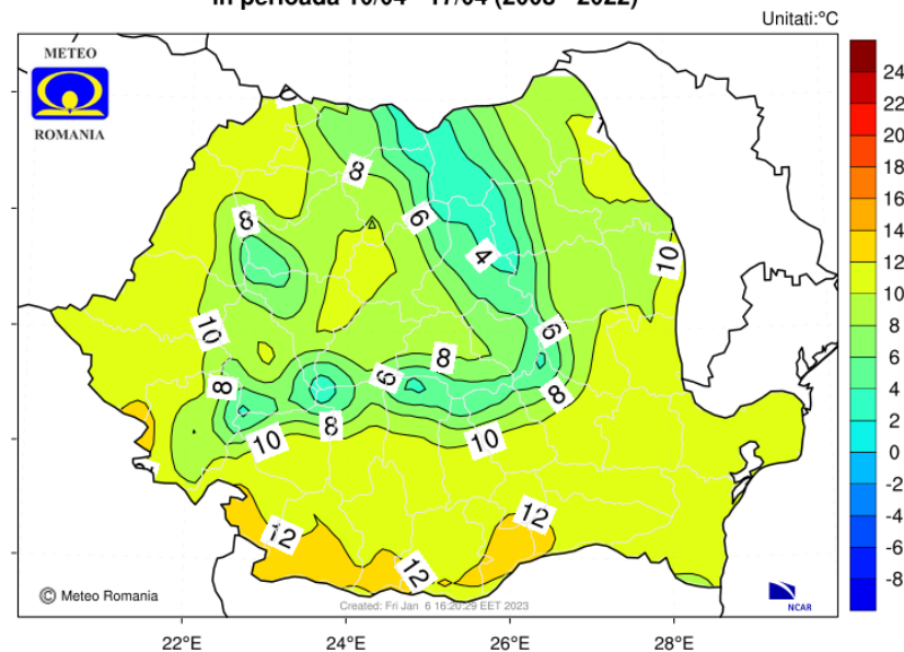
Media multianuala a temperaturii aerului la 2 m in perioada 10/04 - 17/04 (2003 - 2022)
