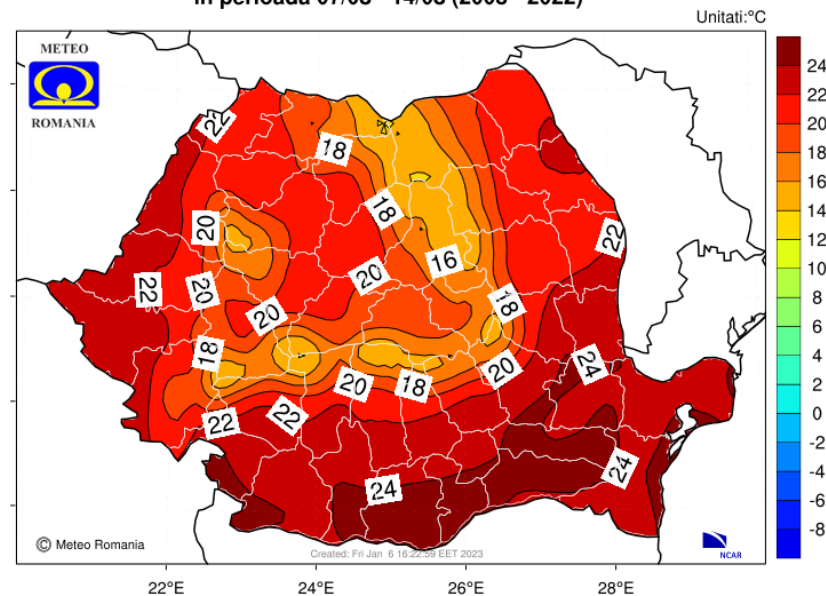
Media multianuala a temperaturii aerului la 2 m in perioada 07/08 - 14/08 (2003 - 2022)
