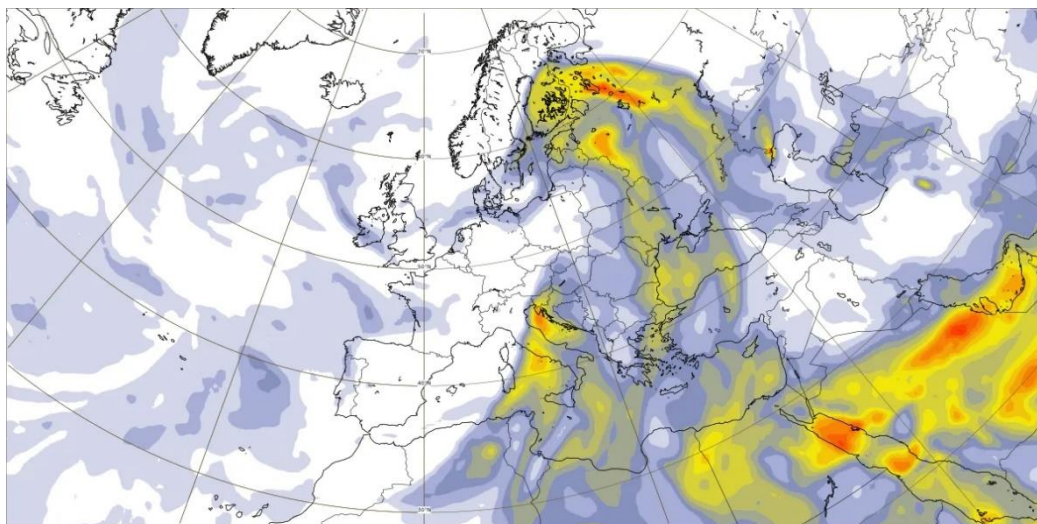
Evoluția masei de aer încărcate cu particule de praf 01 aprilie, ora 12
