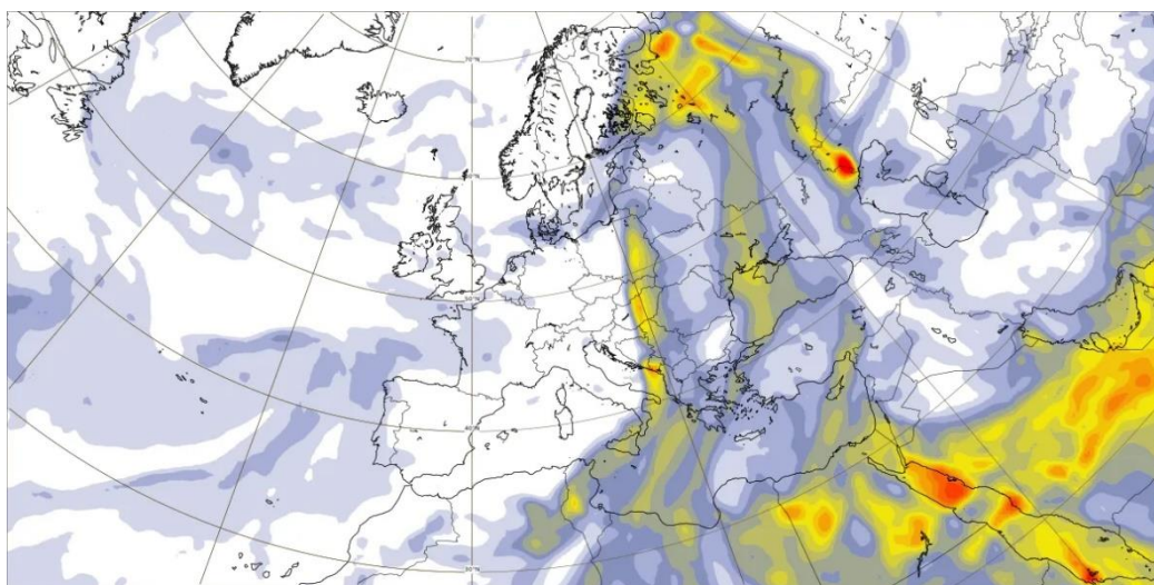
Evoluția masei de aer încărcate cu particule de praf 02 aprilie, ora 00
