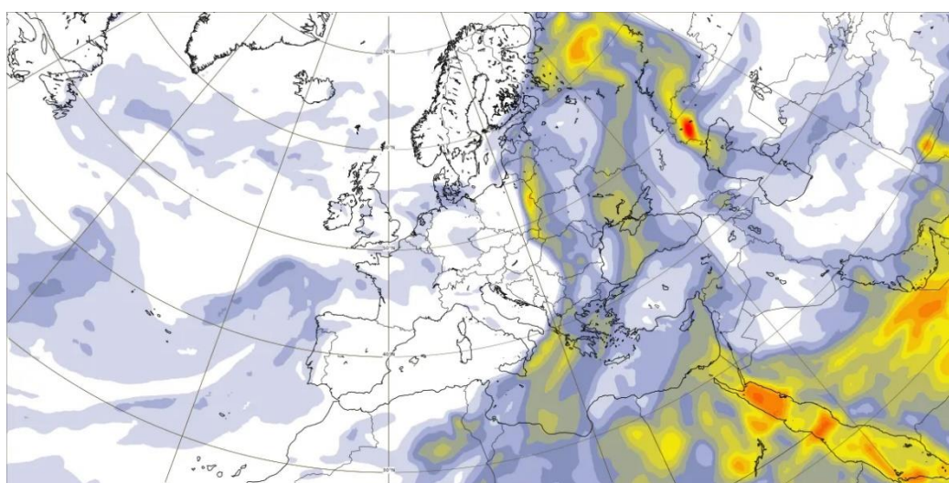
Evoluția masei de aer încărcate cu particule de praf 02 aprilie, ora 06
