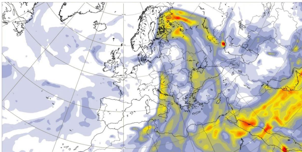
Evoluția masei de aer încărcate cu particule de praf 01 aprilie, ora 18
