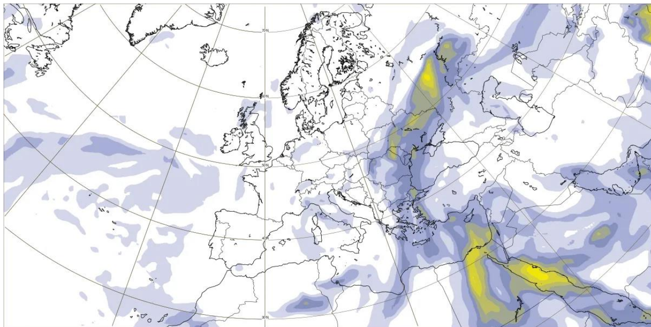
Evoluția masei de aer încărcate cu particule de praf 22 noiembrie, ora 00
