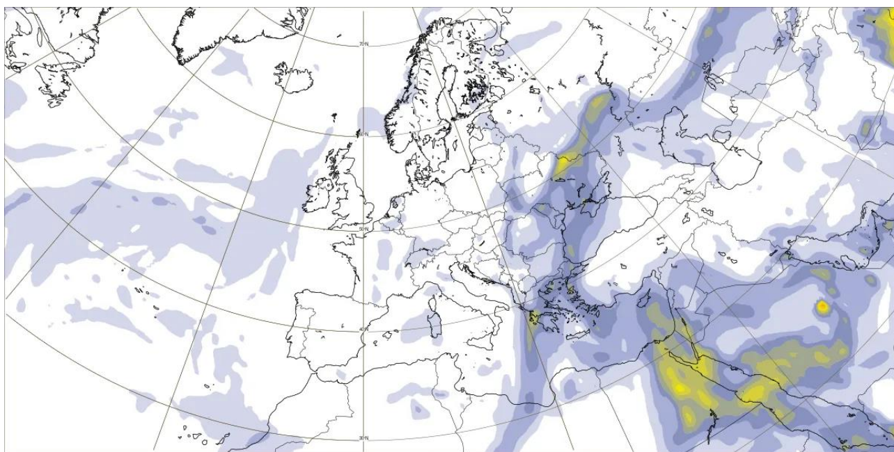
Evoluția masei de aer încărcate cu particule de praf 21 noiembrie, ora 12
