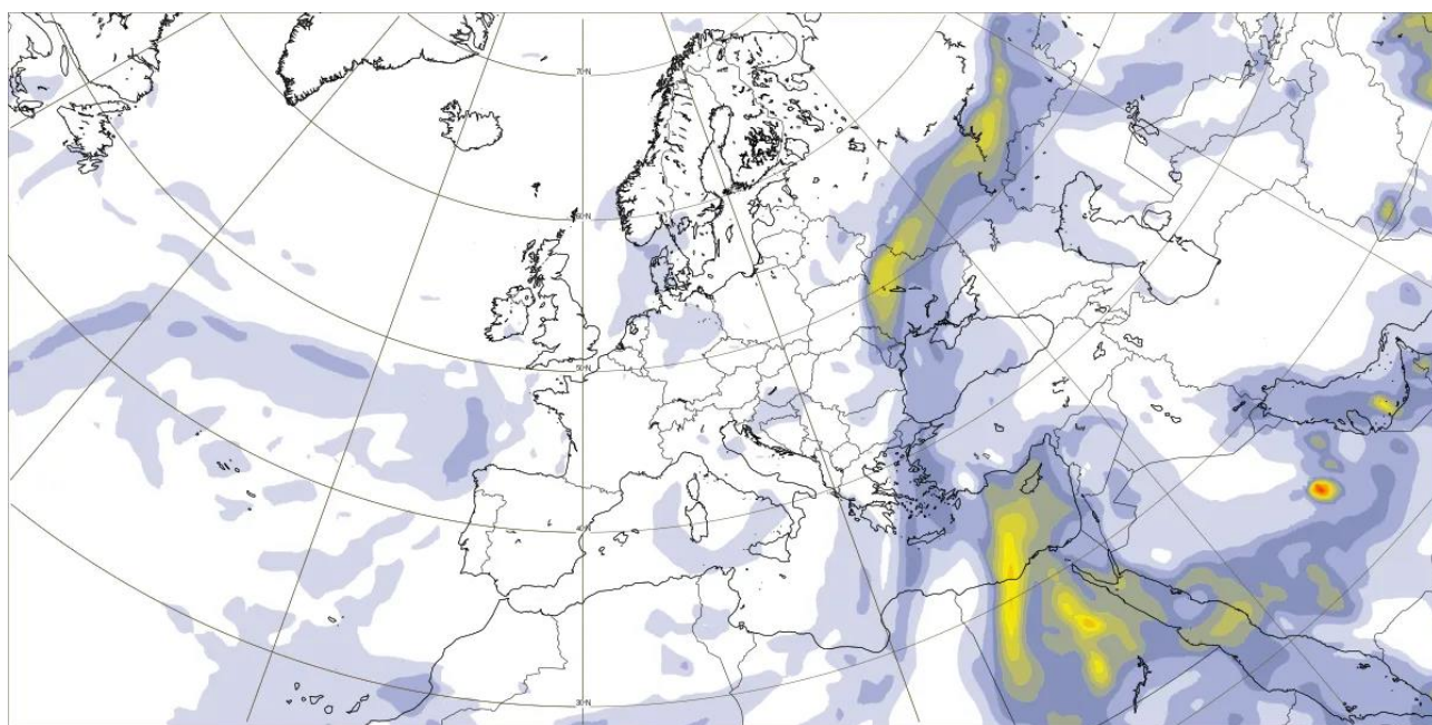
Evoluția masei de aer încărcate cu particule de praf 22 noiembrie, ora 12
