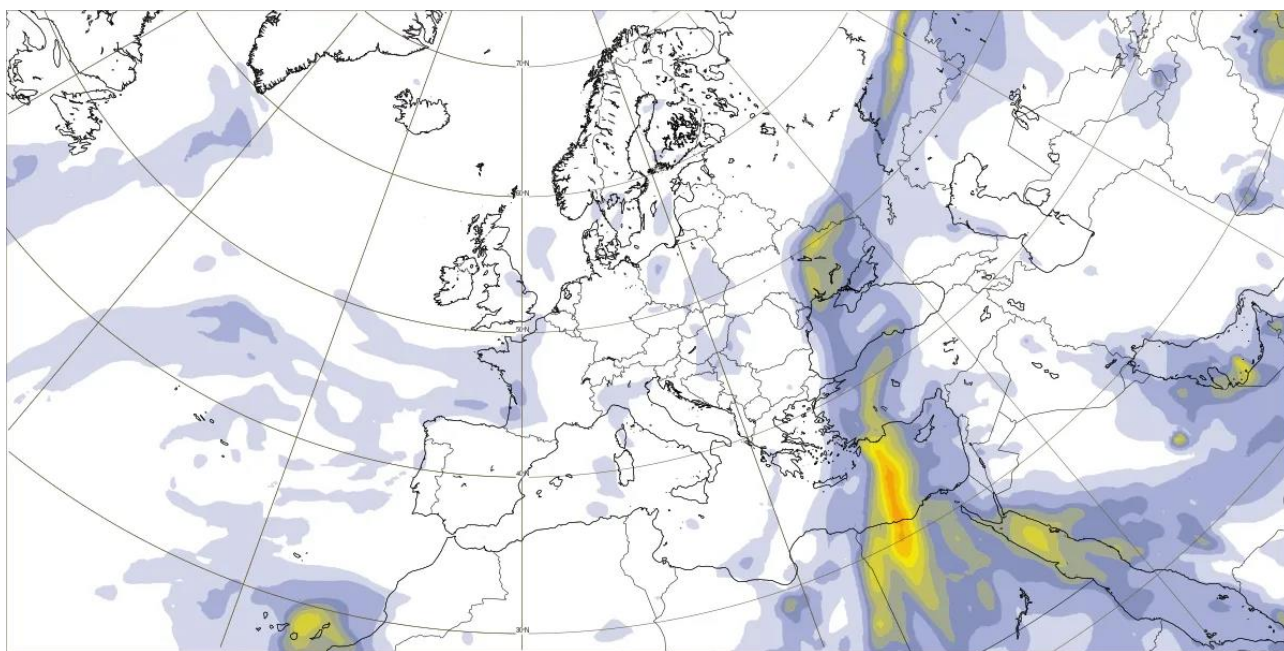
Evoluția masei de aer încărcate cu particule de praf 23 noiembrie, ora 12
