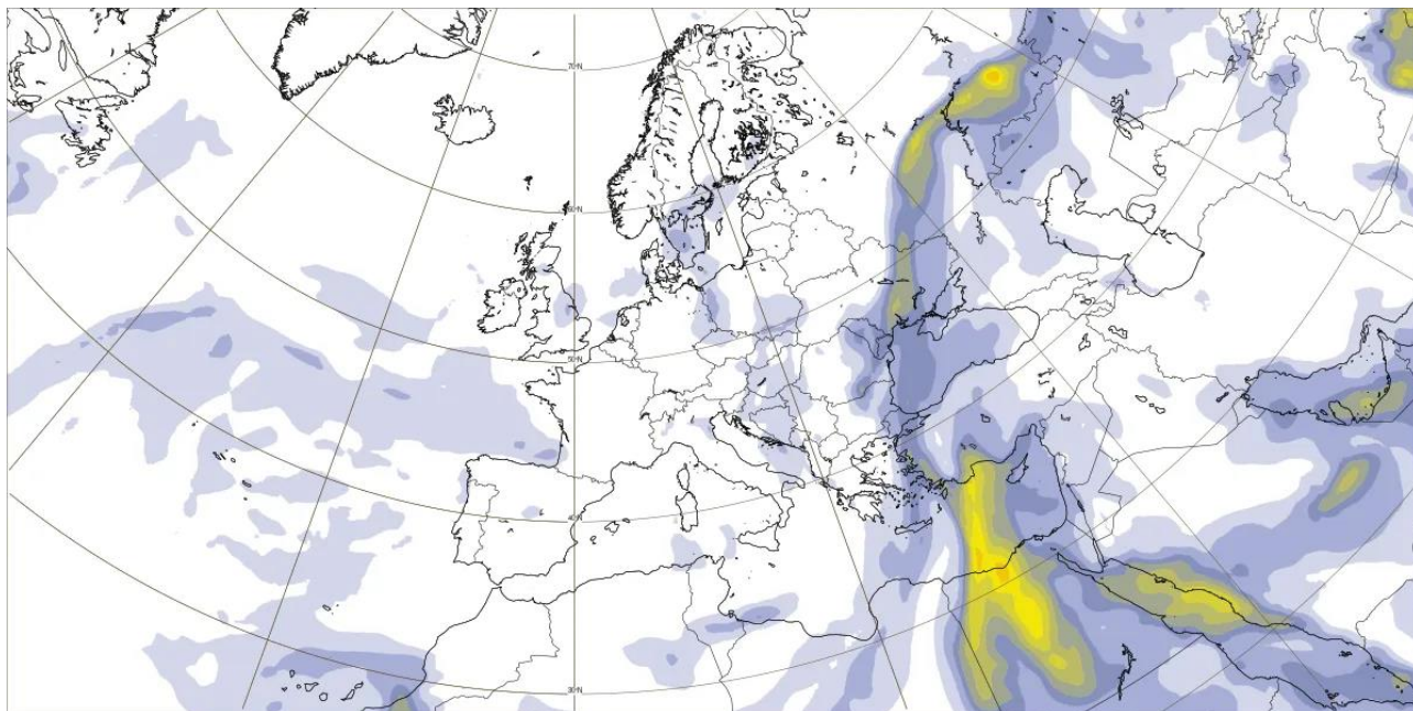
Evoluția masei de aer încărcate cu particule de praf 23 noiembrie, ora 00
