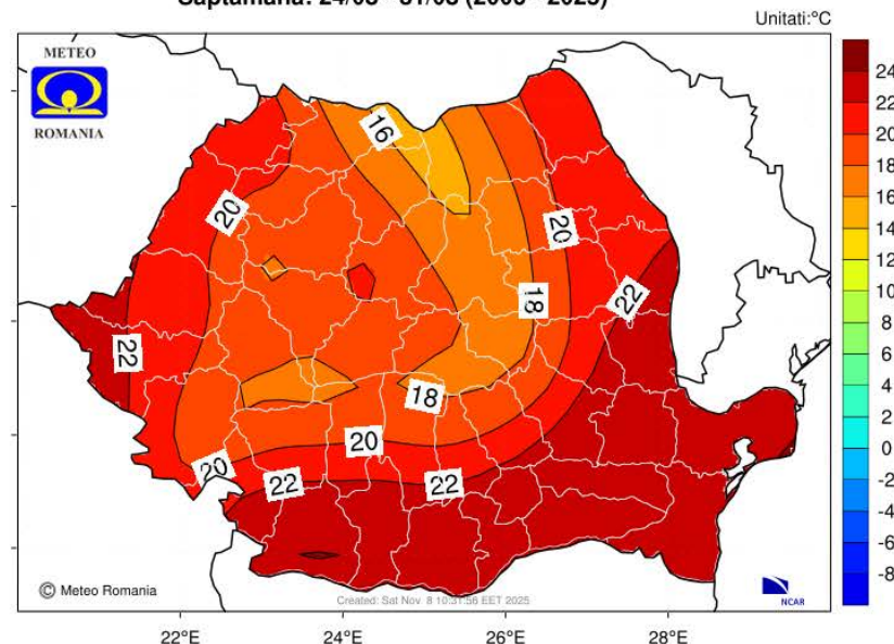
Media multianuala a temperaturii aerului la 2 m Saptamana: 24/08 - 31/08 (2006 - 2025)
