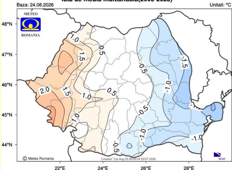
Abaterea temperaturii medii a aerului in perioada 24/08/2026 - 31/08/2026 fata de media multianuala(2006-2025)
